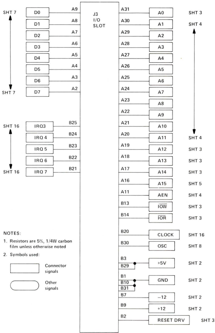
I/O Slot J3
